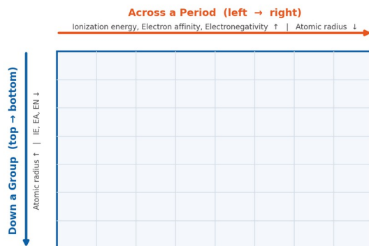
Periodic Trends in the Periodic Table
